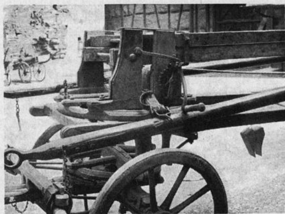
Drehscheibe und Ausziehwinde der Drehleiter, erfunden von dem Tüftler Andreas Scheck in Lienzingen Anno 1808
